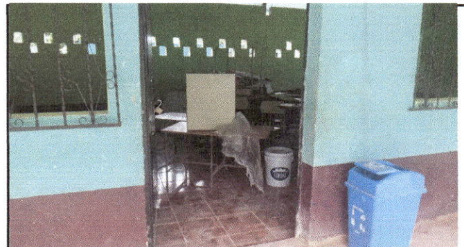
Foto 6: instalación de piso cerámico en el aula No.1 del módulo 2.
