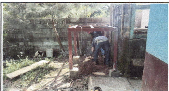
Foto 12: instalación de base de depósito de agua No.2 (tinaco)
